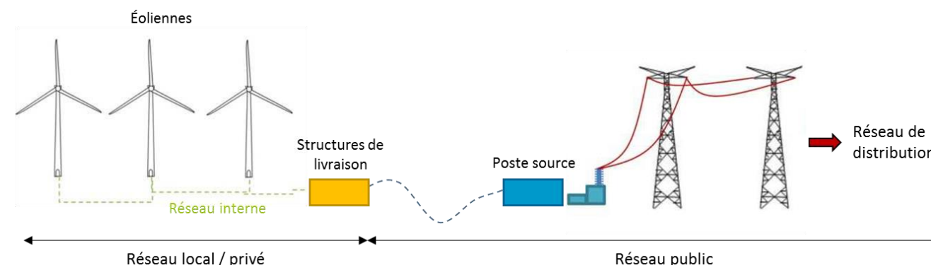
Figure 12 : Schéma de principe de raccordement du parc éolien au réseau public (Source : d'après Guide technique de l'étude de dangers, SER-FEE-ENERIS, 2012)
