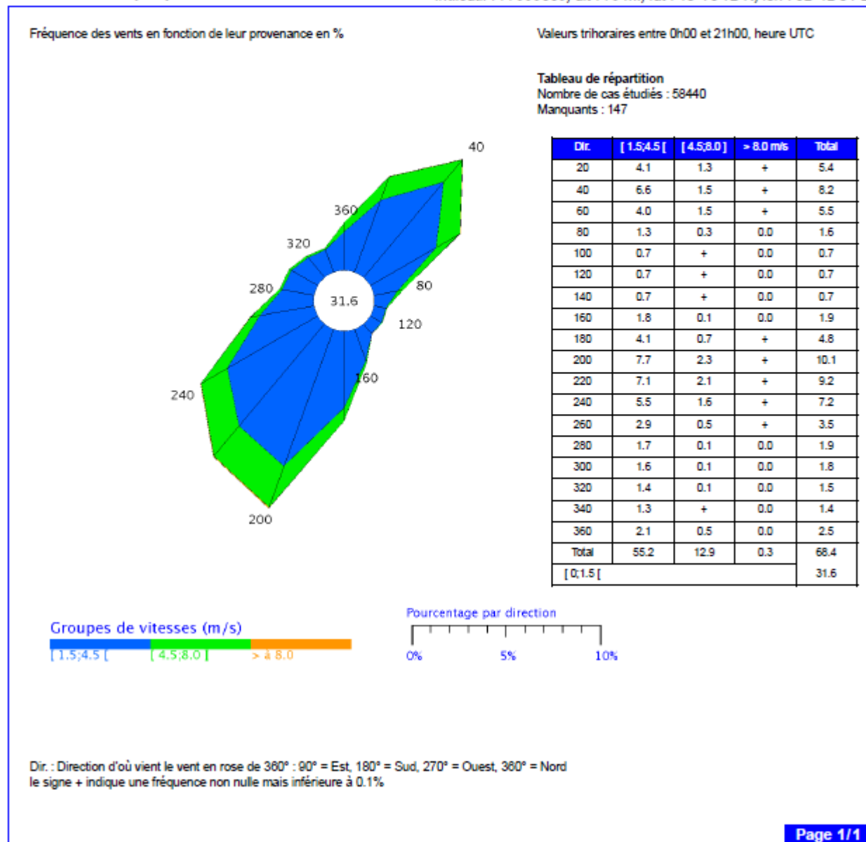
Figure 2 : Rose des vents à Nemours (77) de 1991 à 2010 (Source : Météo France)
