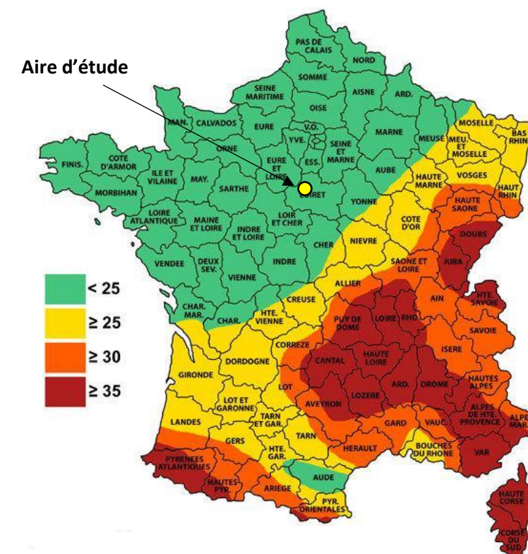
Figure 5 : Niveau kéraunique en France (nombre de jours d'orage par an)
