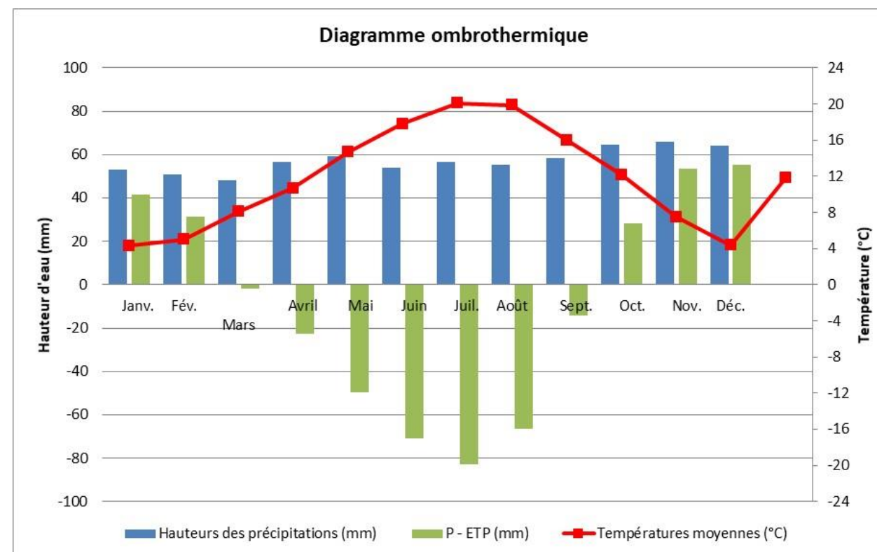
Figure 1 : Diagramme ombrothermique (hauteur d'eau et température) à Nemours entre 1990 et 2010
